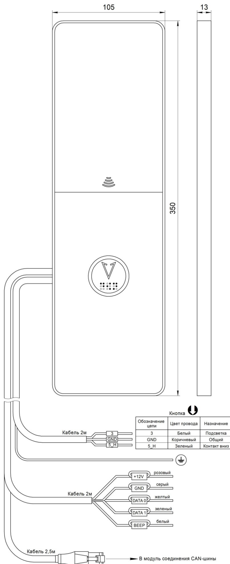
Рис.1 Внешний вид, габаритные и установочные размеры Вызывного поста МАЛАХИТ (жгут RJ45) НШЕК.468381.015-19
